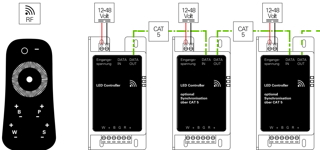
Ausgänge für LED-Stripes/Leuchten
