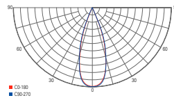
36° Standard-Abstrahlwinkel mit 36°-Linse [Standard]
