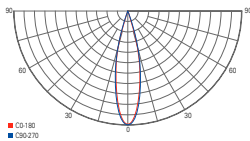
24° Enger Abstrahlwinkel mit optionaler 24°-Linse
